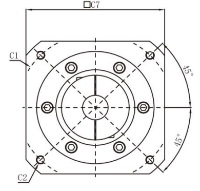
输入端/INPUT
